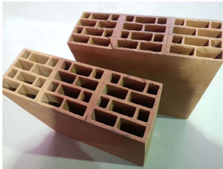
Abb. 1: Der modifizierte Ziegel (unten) hat im unporierten Zustand eine höhere Festigkeit bei gleicher WLF. Er kann also stärker poriert werden, wodurch sich eine niedrigere WLF erzielen lässt.
